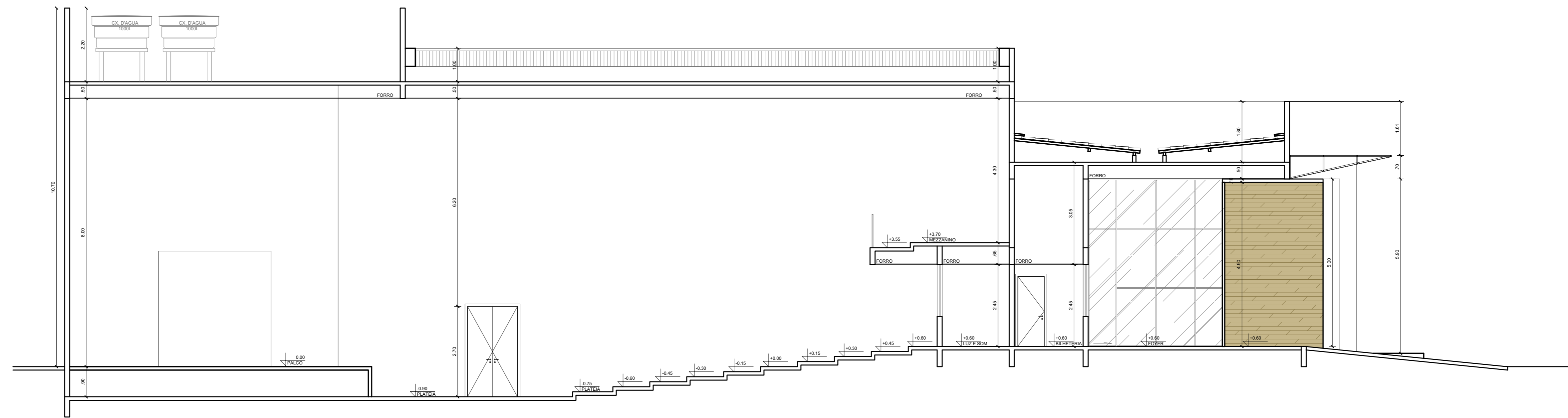
CORTE BB' ESC 1/75
