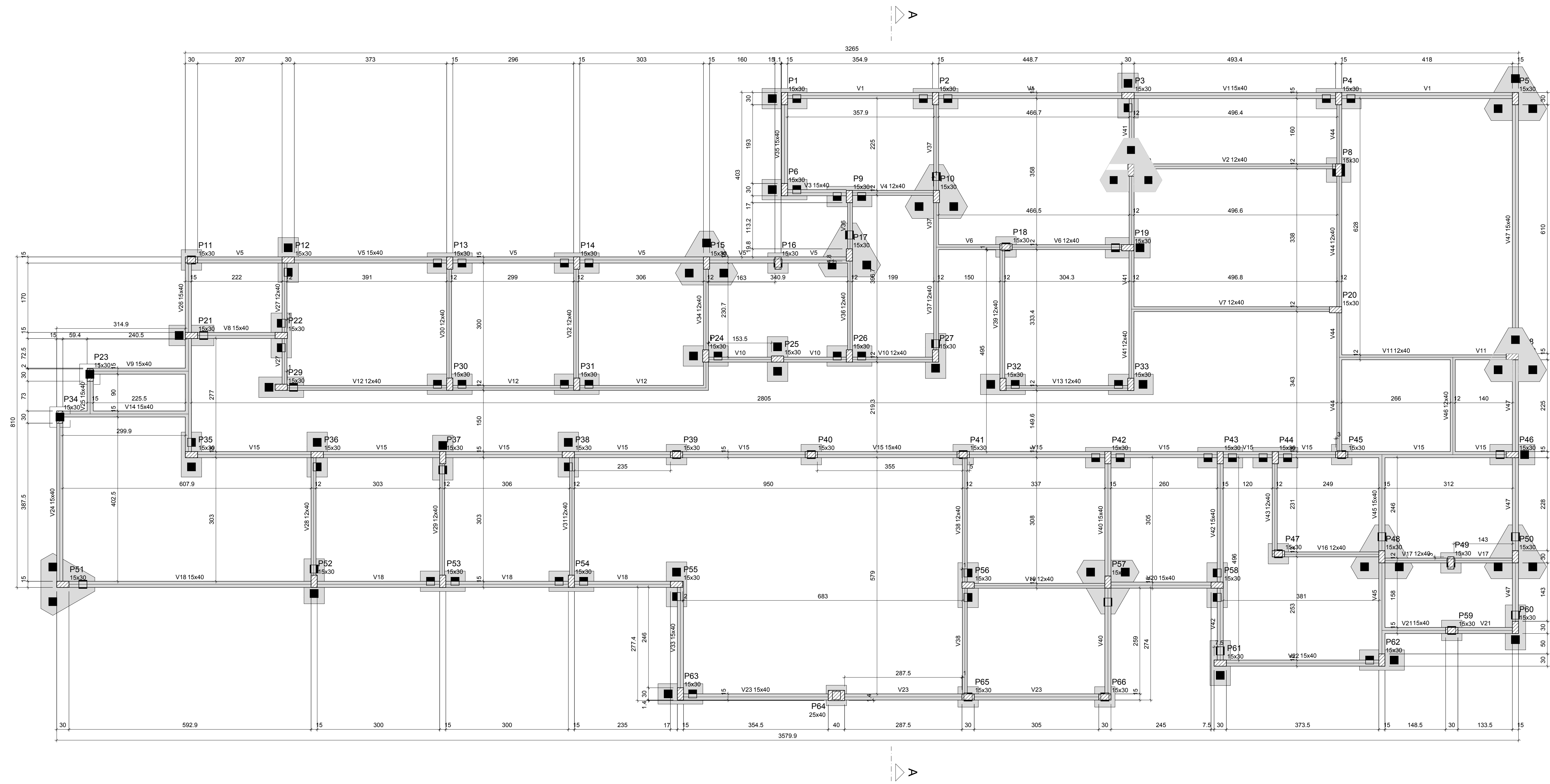
Forma do pavimento FUNDAÇÃO escala 1:50
