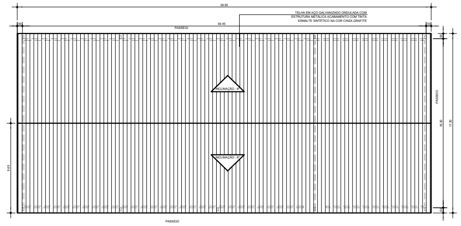
PLANTA DE COBERTURA ESC. 1:100
