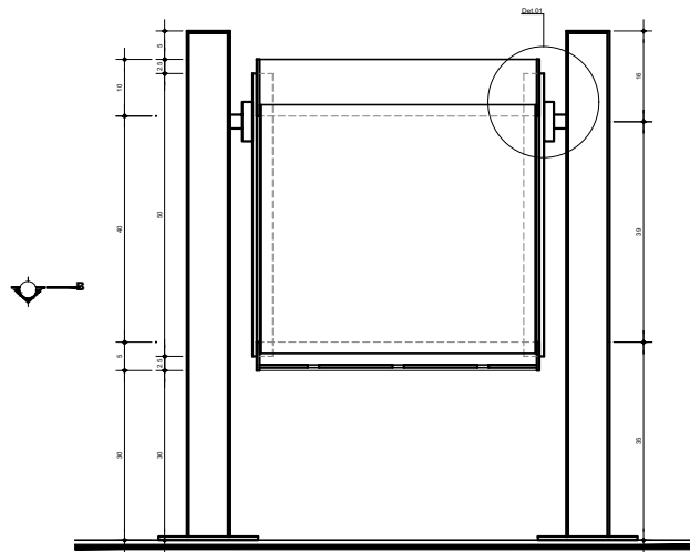
SECÇÃO A ESC. 1:5
