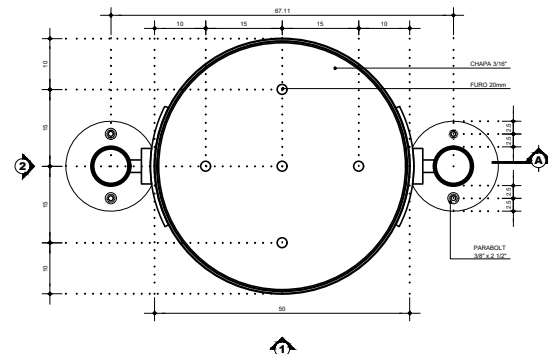
SECÇÃO B COTAS DOS FUROS - ESC. 1:5
