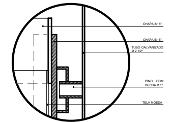
Det.01 ESC. 1:2
