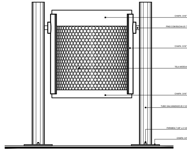
ELEVAÇÃO 1 ESC. 1:5
