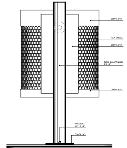
ELEVAÇÃO 2 ESC. 1:5
