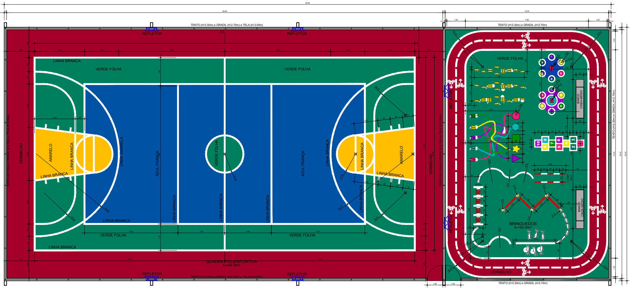
PLANTA BAIXA - PINTURA - QUADRA E BRINQUEDO ESC. 1:50
