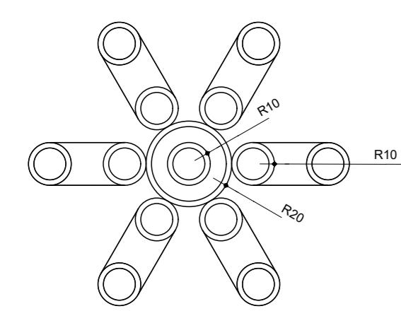
PILAR - PLANTA BAIXA ESC. 1:25
