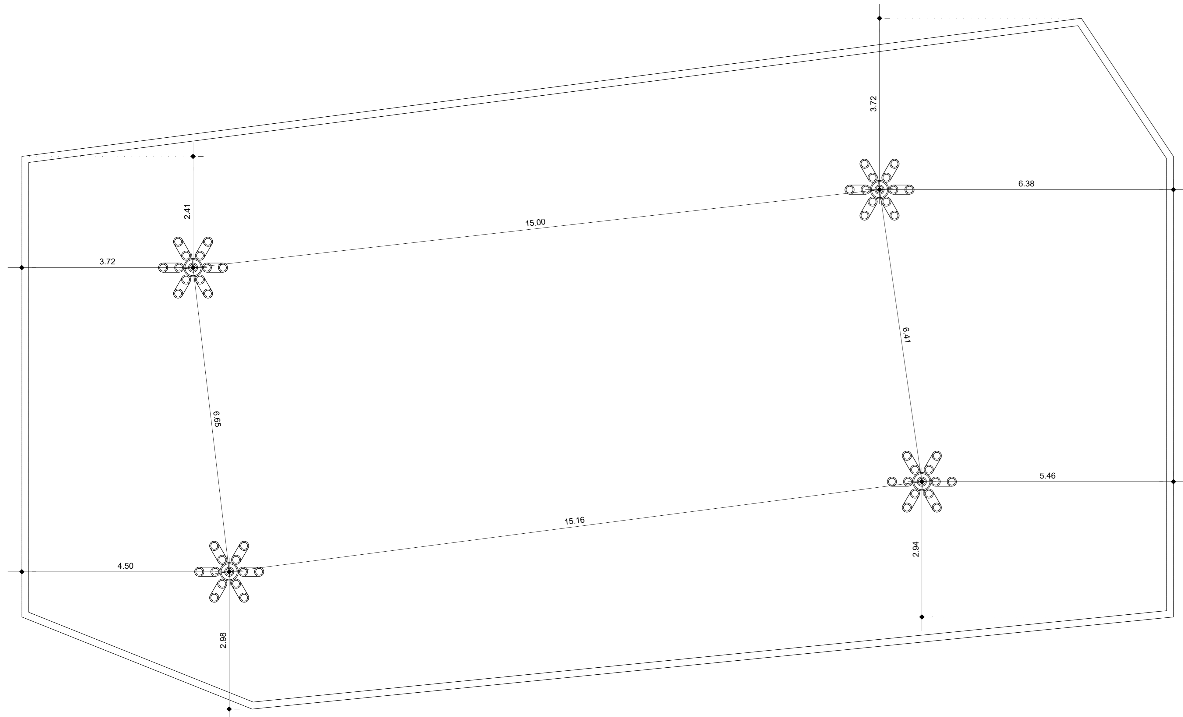
PLANTA BAIXA - ESP. MULTIUSO ESC. 1:75
