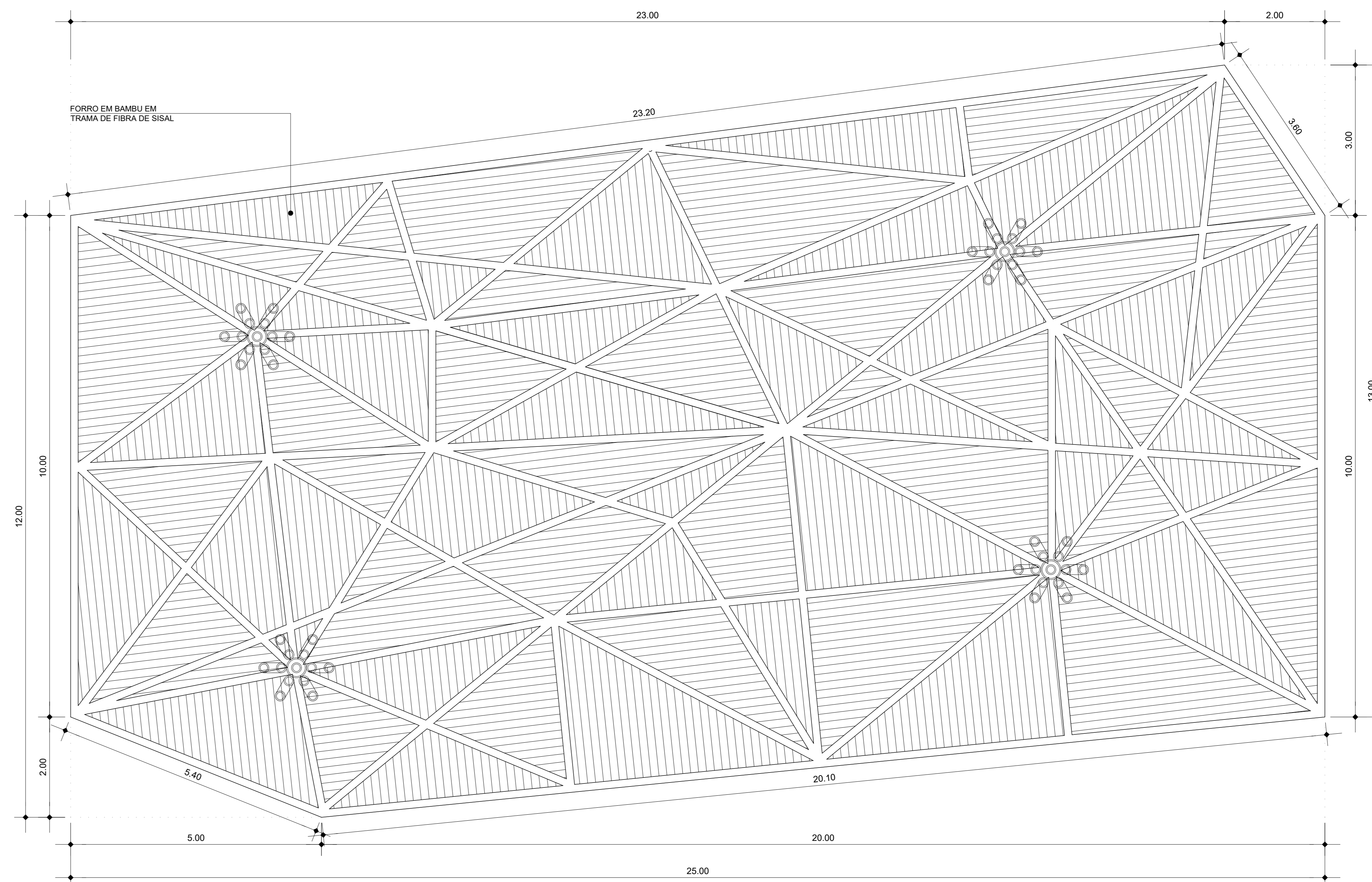
ESTRUTURA MOSAICO - ESP. MULTIUSO ESC. 1:75
