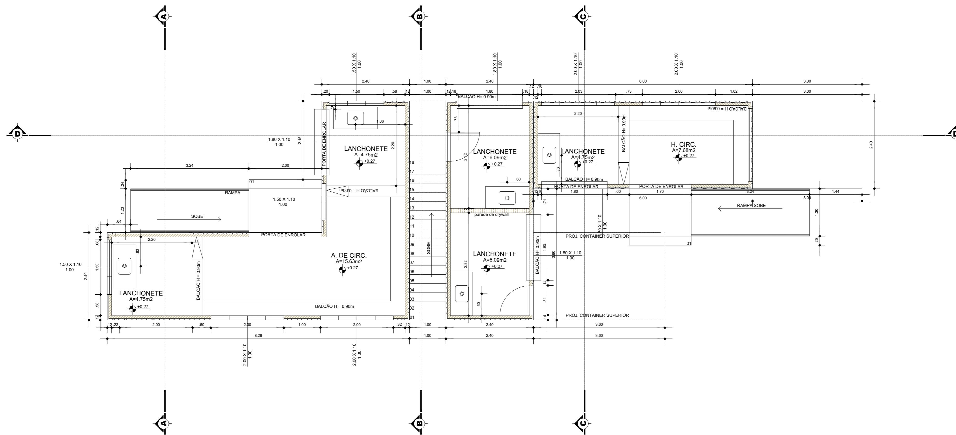
PLANTA BAIXA - TÉRREO (QUIÓSQUE TIPO 01) ESC. 1:50
