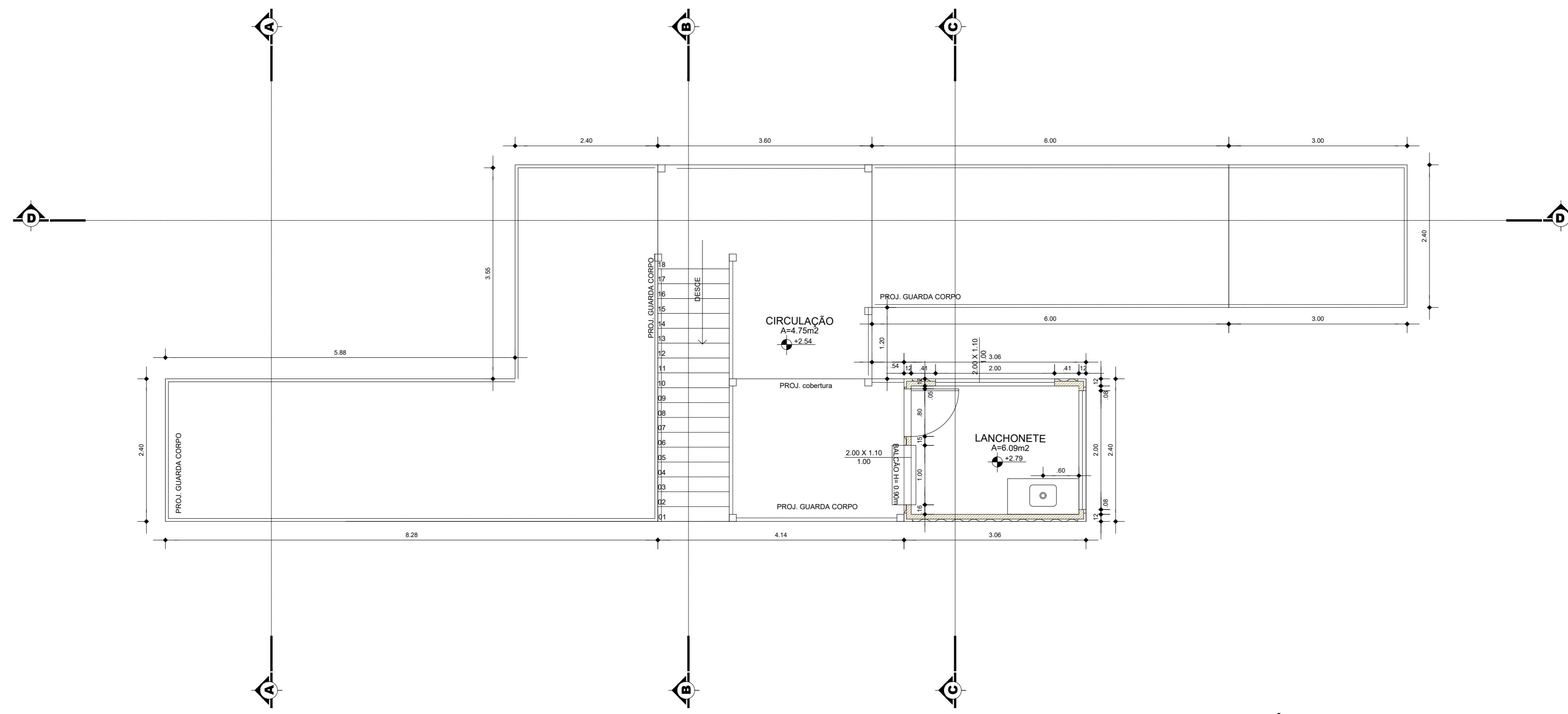
PLANTA BAIXA - SUPERIOR (QUIÓSCUE TIPO 01) ESC. 1:50
