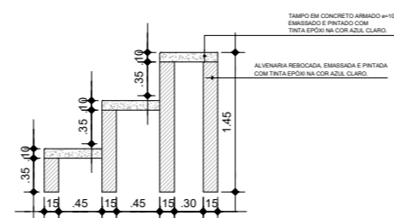
SECÇÃO A - 03 ESC. 1:50
