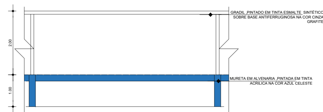
DET 01 ESC. 1:50
