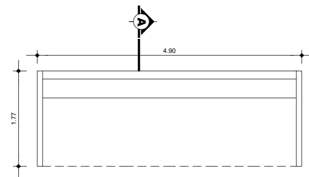
PLANTA BAIXA - DET 02 ESC. 1:50
