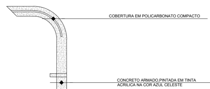
SECÇÃO A - DET 02 ESC. 1:50
