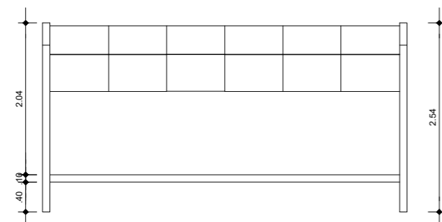
ELEVAÇÃO 1 - DET 02 ESC. 1:50
