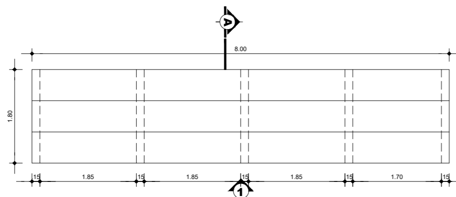
PLANTA BAIXA - DET 03 ESC. 1:50
