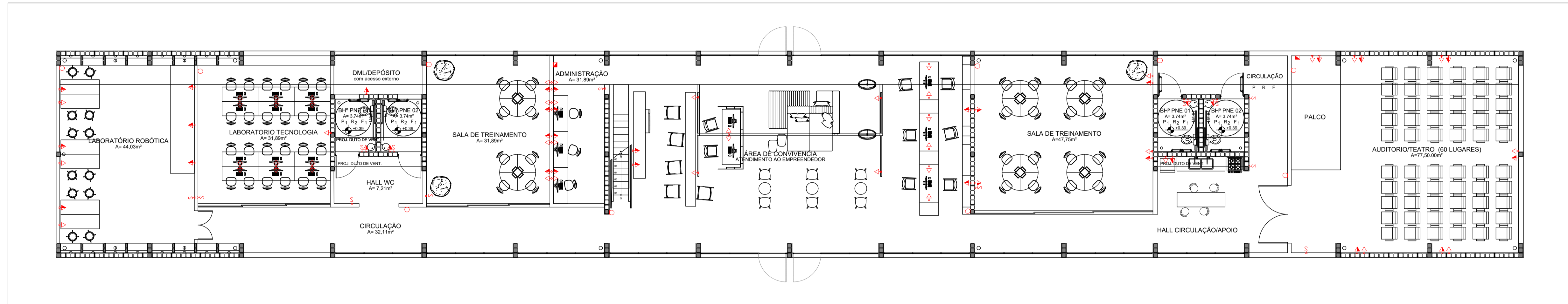
PLANTA PONTOS ELÉTRICOS e HIDRAULICOS - PAV. TÉRREO ESC. 1/75
