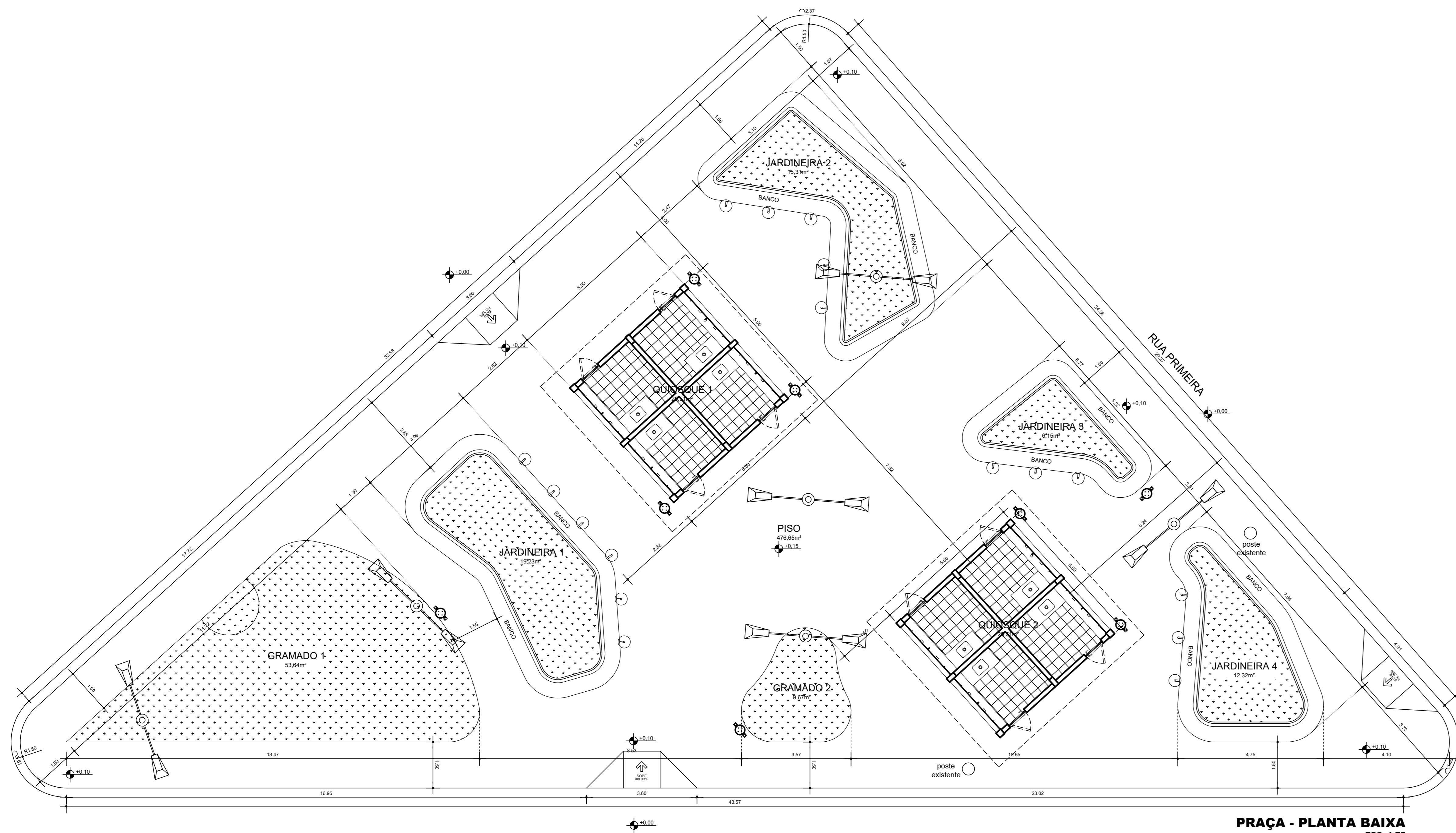
PRAÇA - PLANTA BAIXA ESC. 1:75
