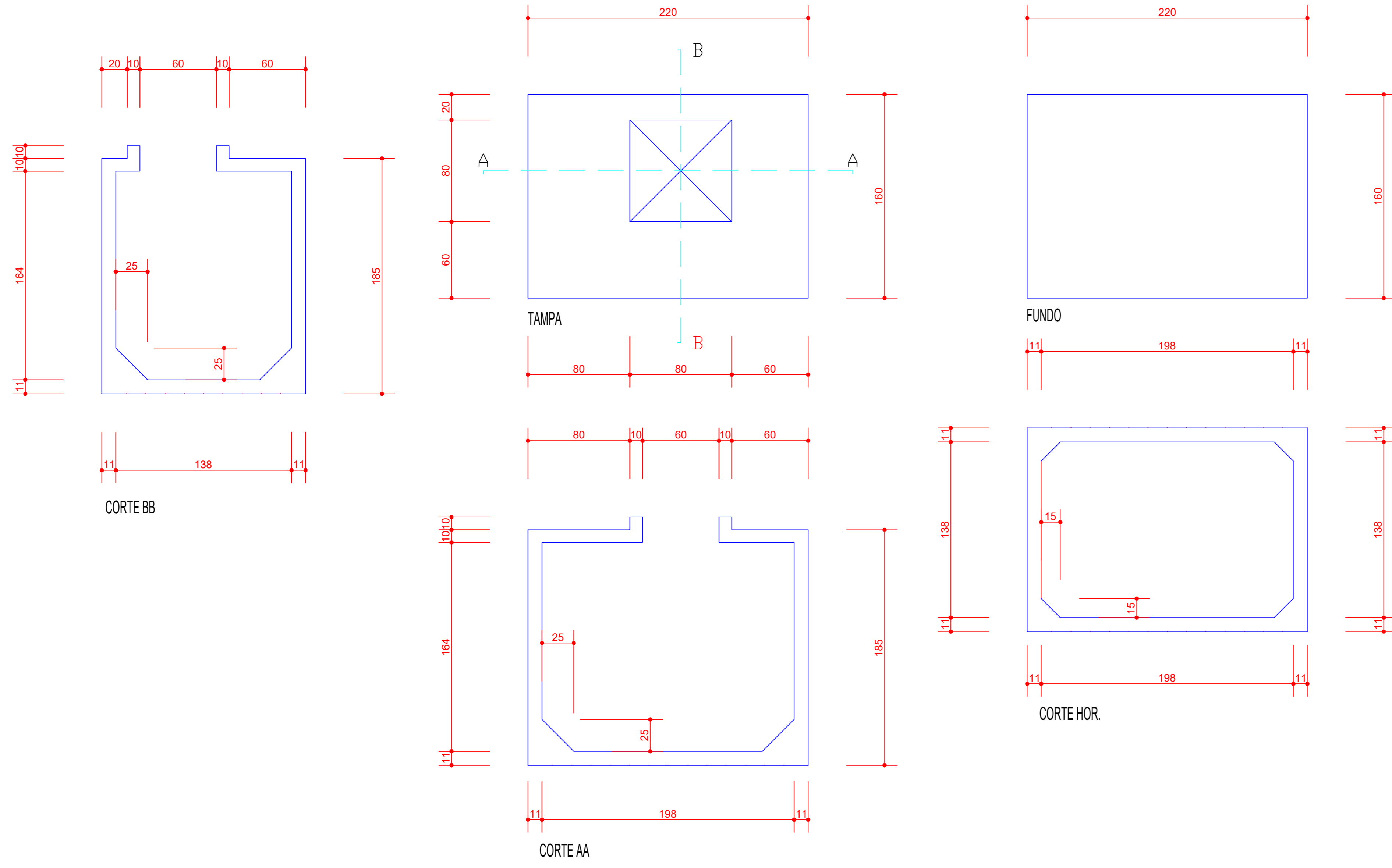
PLANTA: Forma do Corpo do Poço Visita-PV12-SIMPLES-GALERIA "A" - 220x160x185
