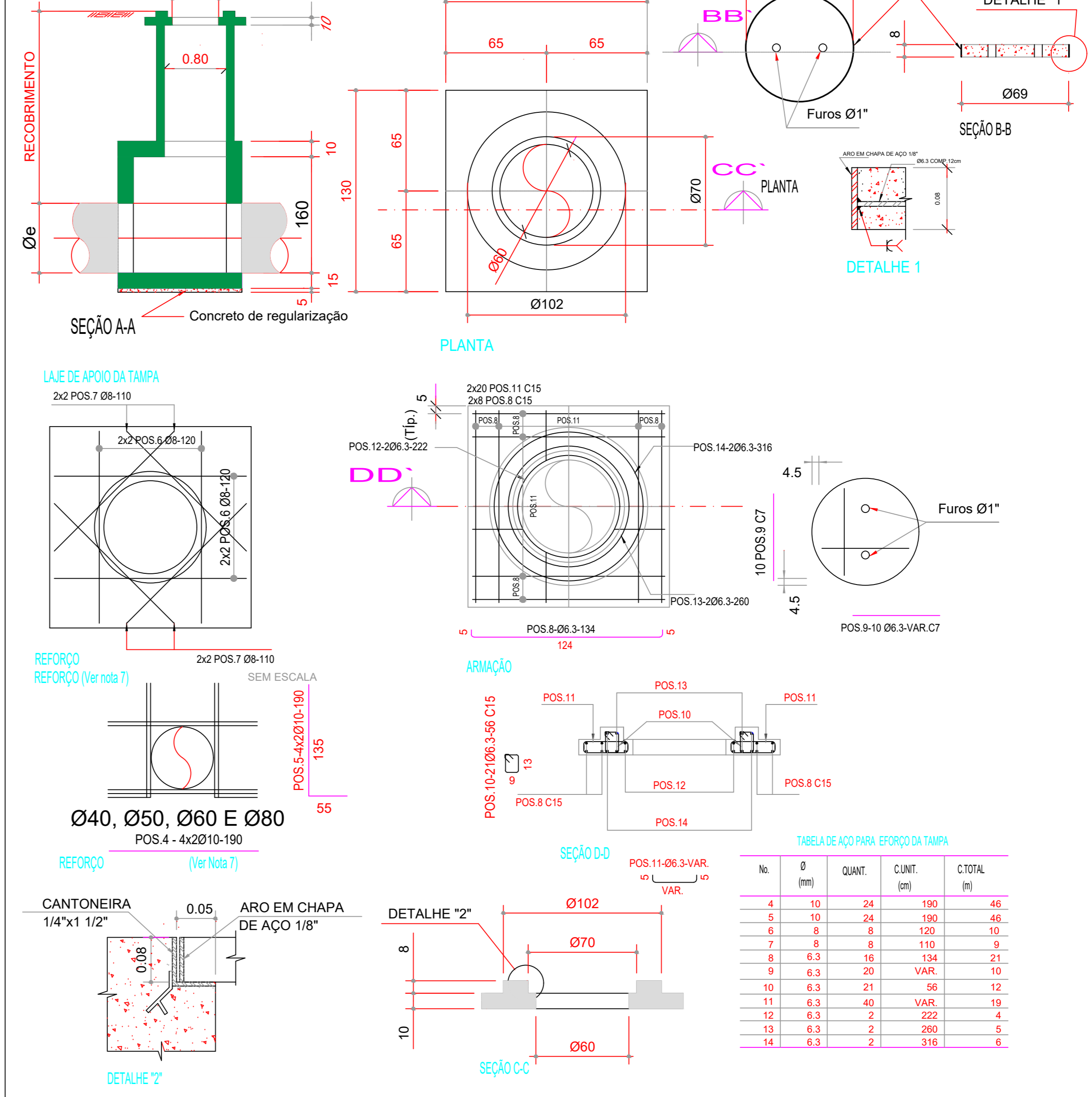
PLANTA: Detalhe da Tampa do Poço Visita-PV3x100-SIMPLES
