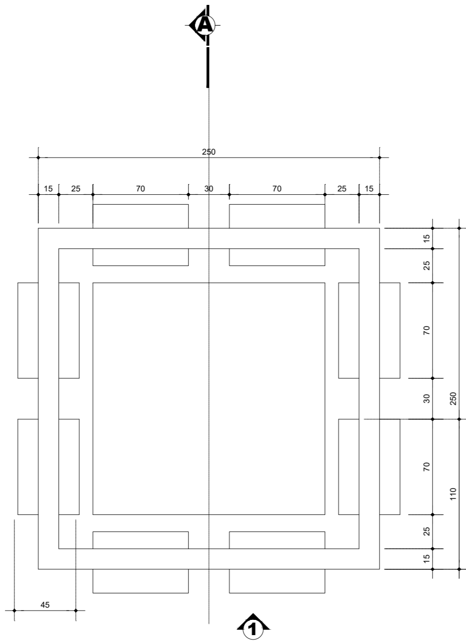
PLANTA BAIXA - MESA COM BALANÇO ESC. 1:25
