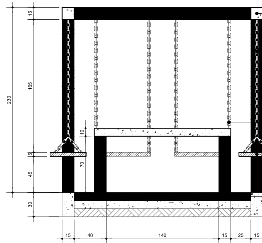
CORTE A- MESA COM BALANÇO ESC. 1:25
