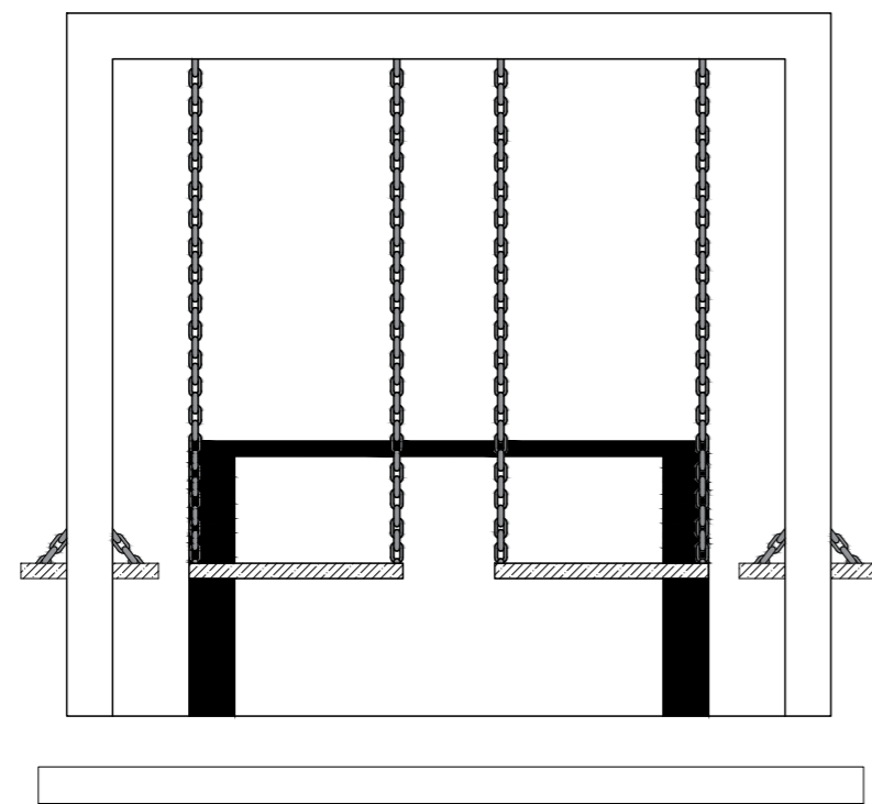
VISTA 1 e 2 - MESA COM BALANÇO ESC. 1:25
