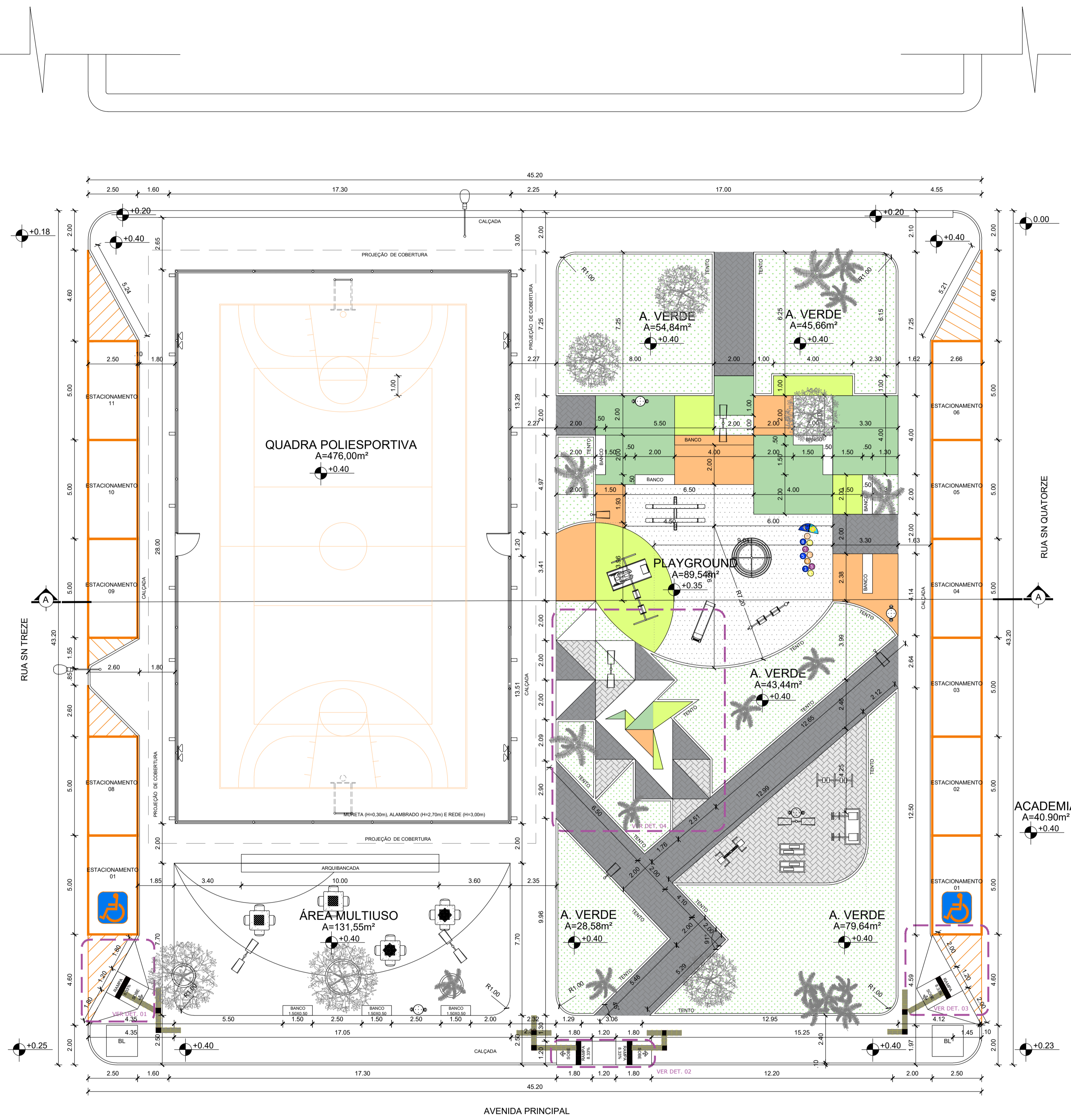
PLANTA BAIXA ESC. 1:125
