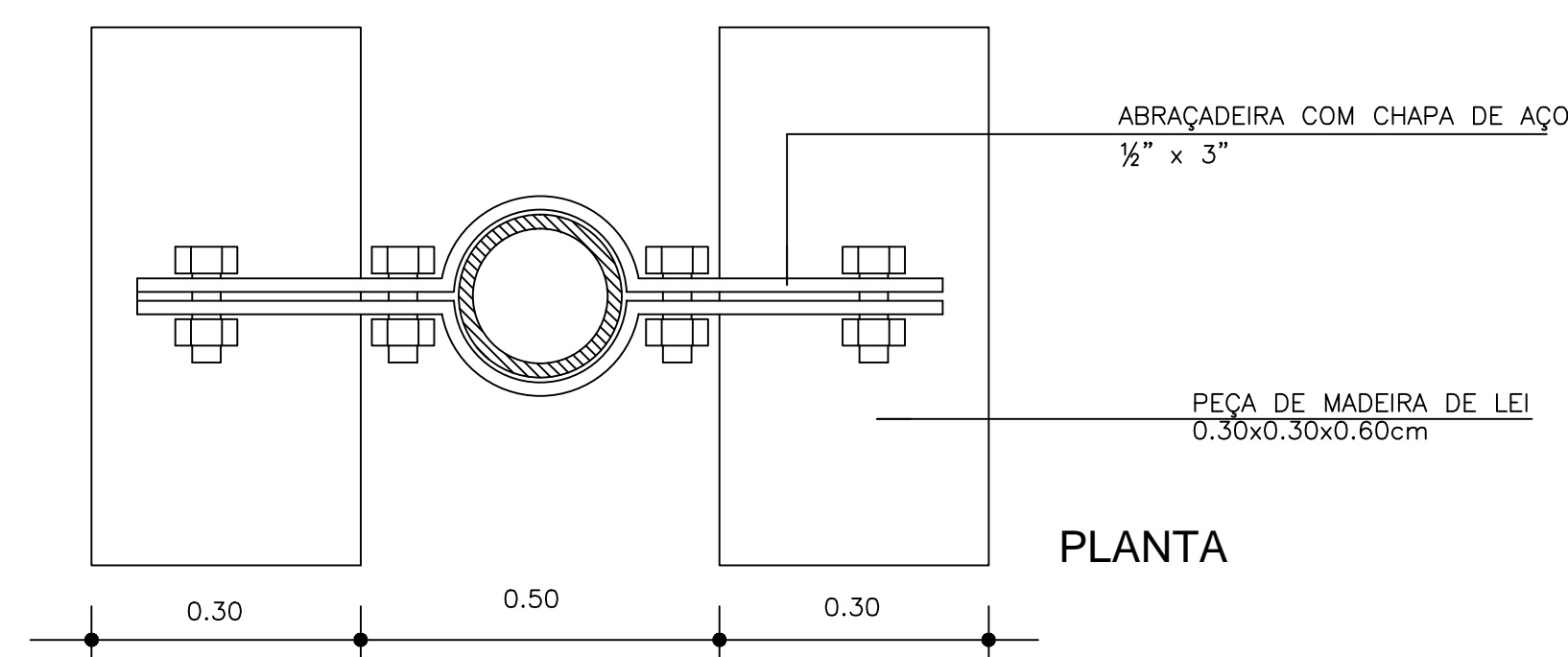
DETALHE - 03 ESCALA 1:10
