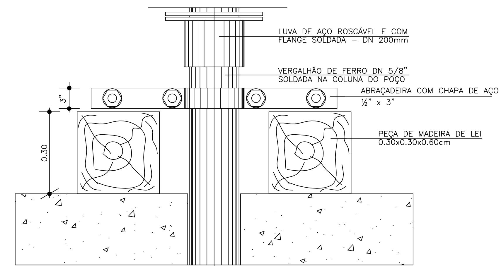
CORTE
