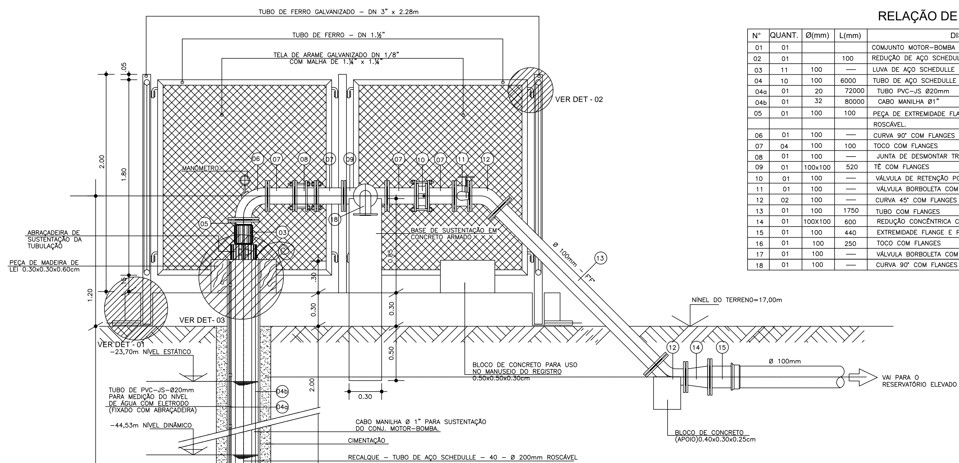
PERFIL DO POÇO E BARRILETE ESCALA 1:20
