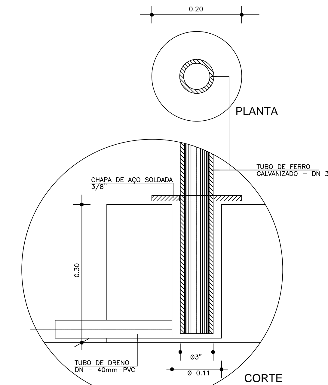
CORTE
