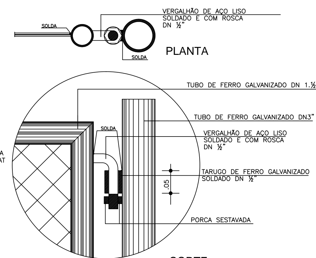
CORTE
