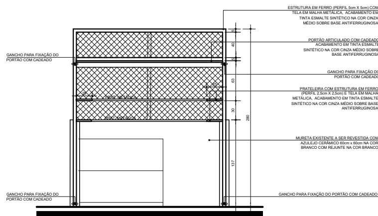
ELEVAÇÃO 1 - HORTIFRUTI/TEMPEROS/FARINHA ESC. 1:25 (PORTÃO ARTICULADO ABERTO)
