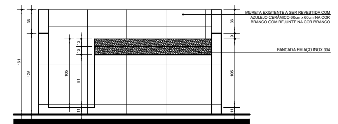
ELEVAÇÃO 1 - PEIXE ESC. 1:25
