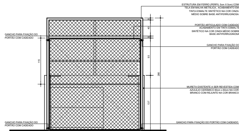
ELEVAÇÃO 1 - HORTIFRUTI/TEMPEROS/FARINHA ESC. 1:25 (PORTÃO ARTICULADO FECHADO)
