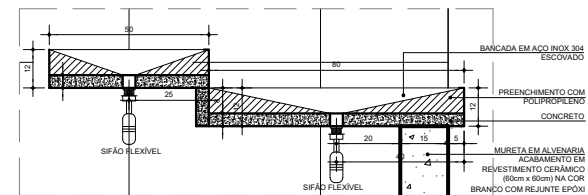
DET.01 - SECÇÃO A - PEIXE ESC. 1:10
