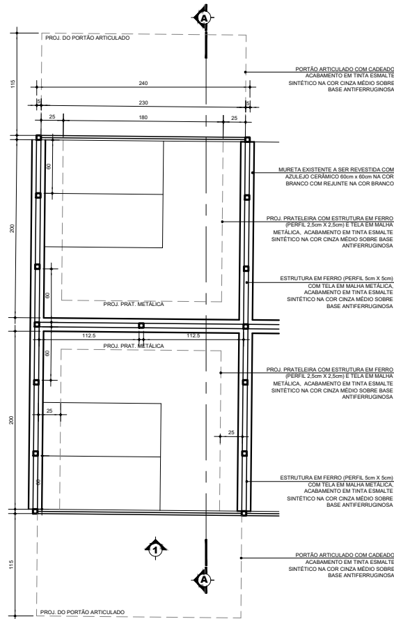
PLANTA BAIXA - HORTIFRUTI/TEMPEROS/FARINHA ESC. 1:25
