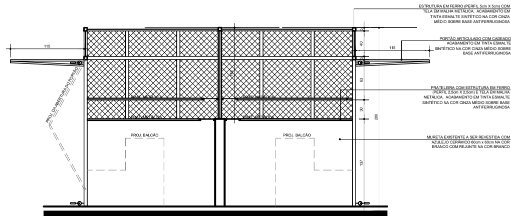
SECÇÃO A - HORTIFRUTI/TEMPEROS/FARINHA ESC. 1:25 (PORTÃO ARTICULADO ABERTO)
