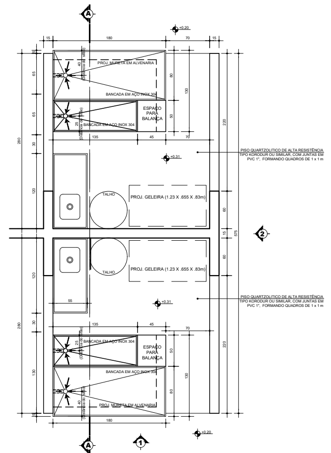
PLANTA BAIXA - PEIXE ESC. 1:25
