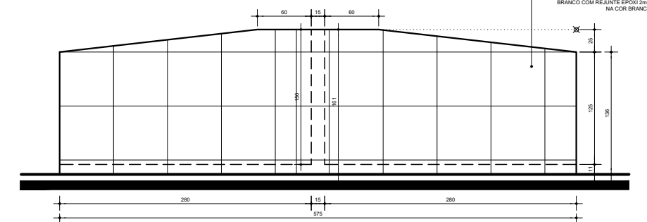
ELEVAÇÃO 2 - PEIXE ESC. 1:25
