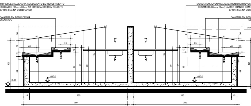
SECÇÃO A - PEIXE ESC. 1:25
