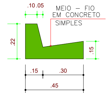
DETALHE-01: SEM ESCALA
