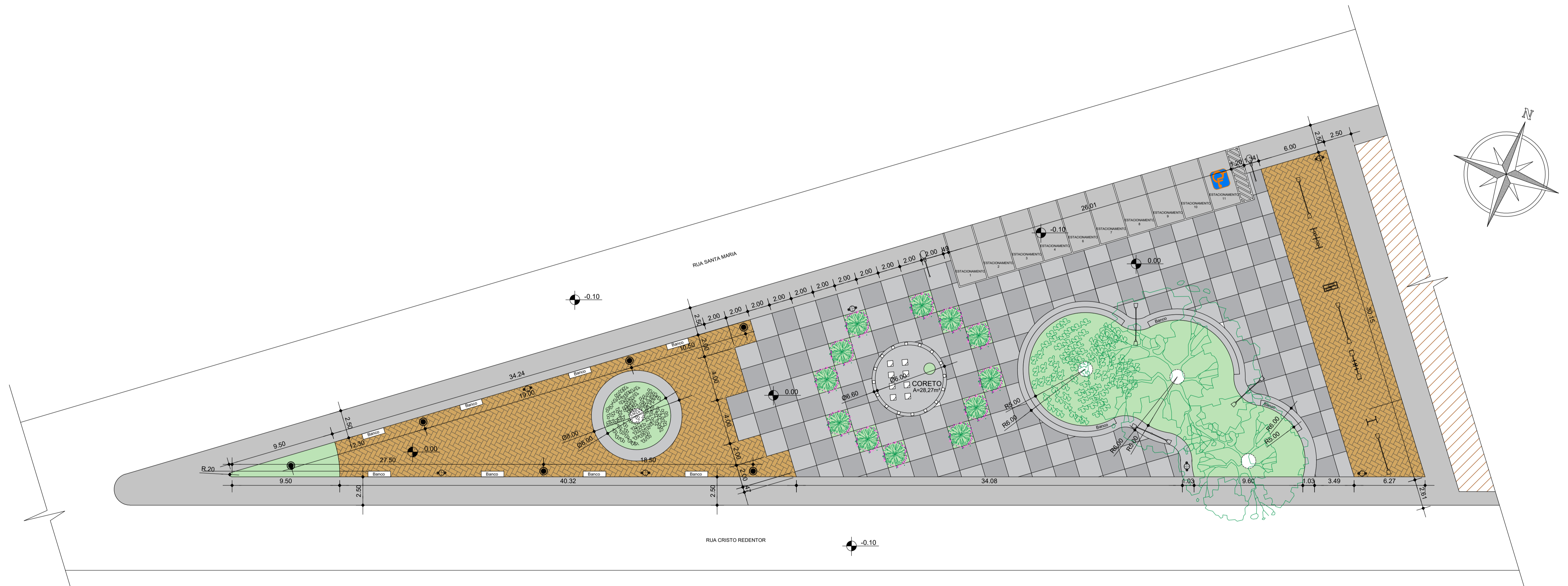
LAYOUT E PAGINAÇÃO DE PISO ESC. 1:200
