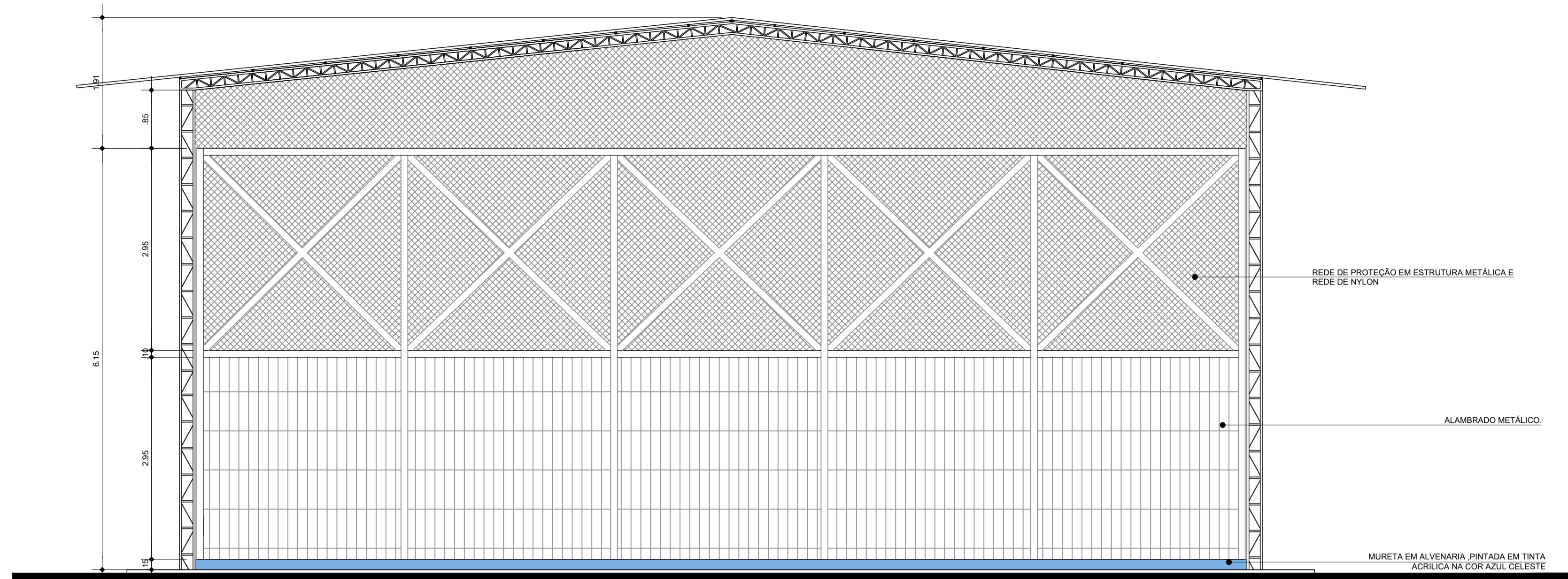
ELEVAÇÃO 1 ESC. 1:50
