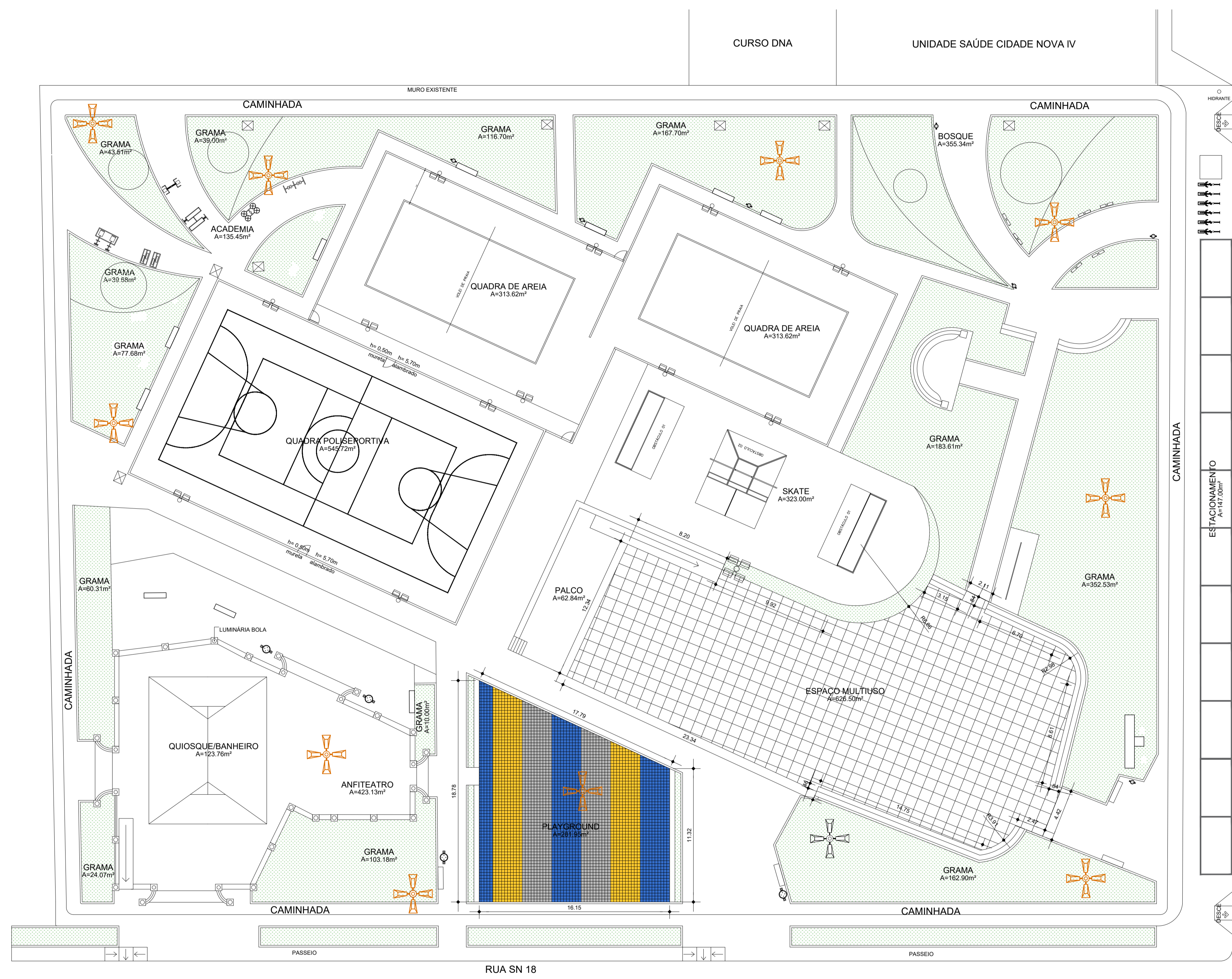
PLANTA BAIXA ESC.: 1:200
