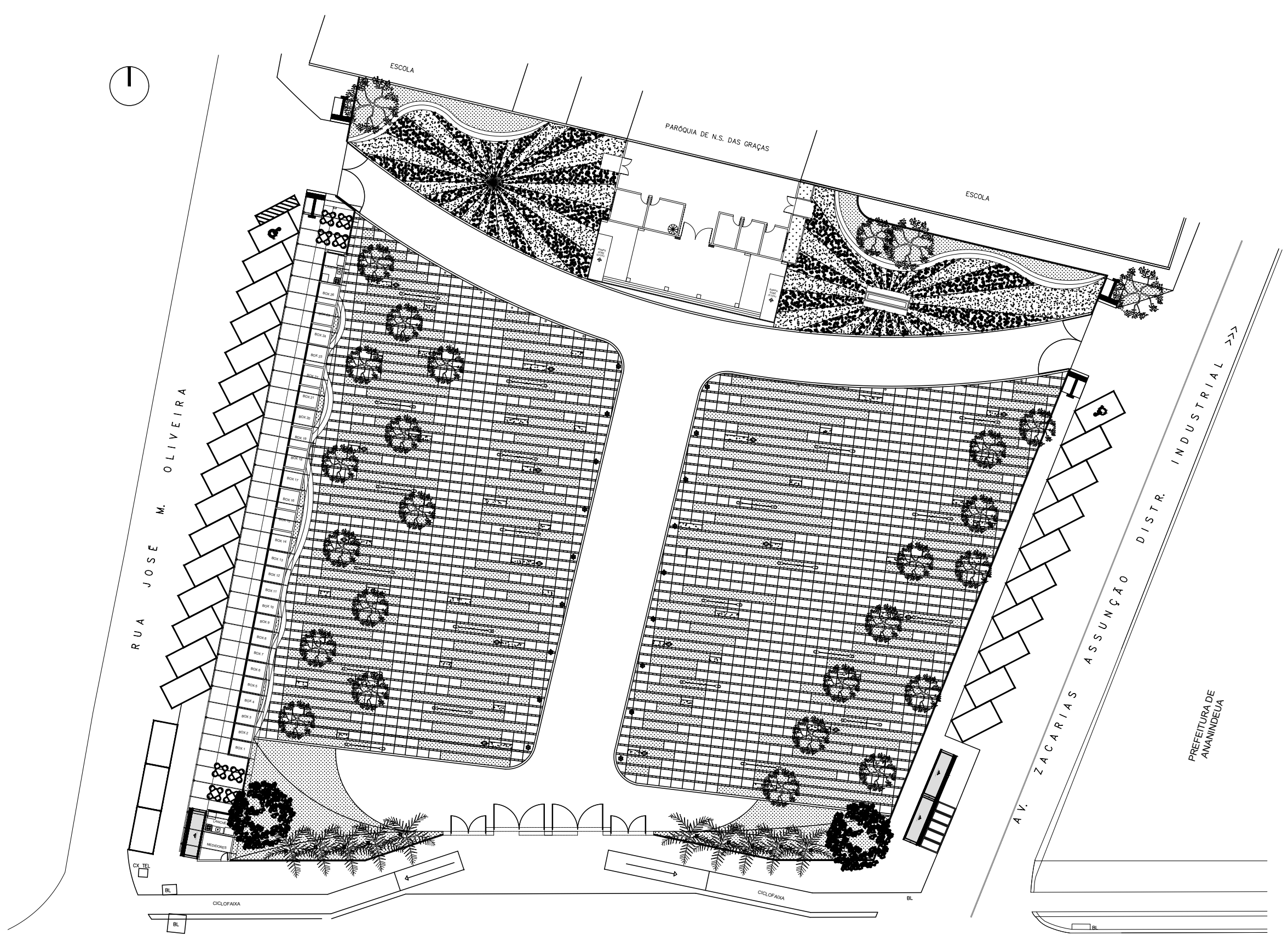
PLANTA DE LAYOUT ESC. 1:150
