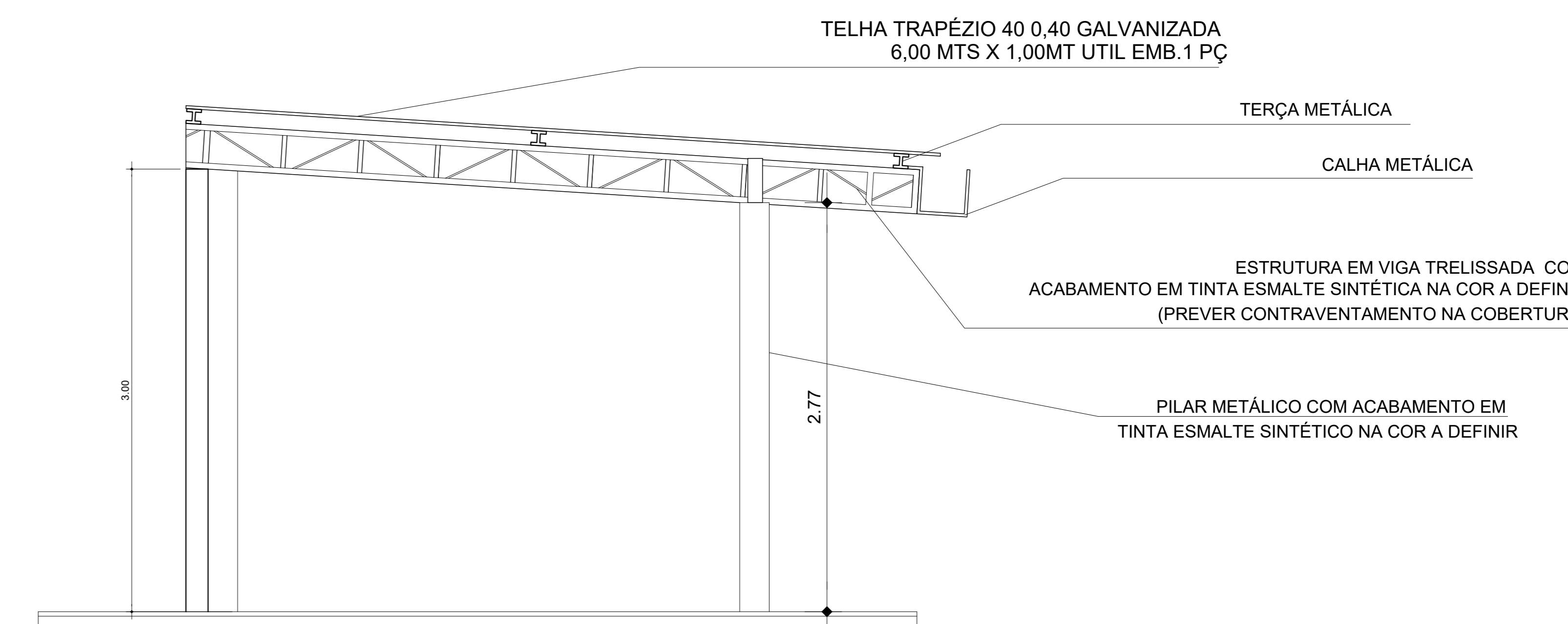
CORTE A - ESPAÇO FOOD TRUCK Esc. 1:25
