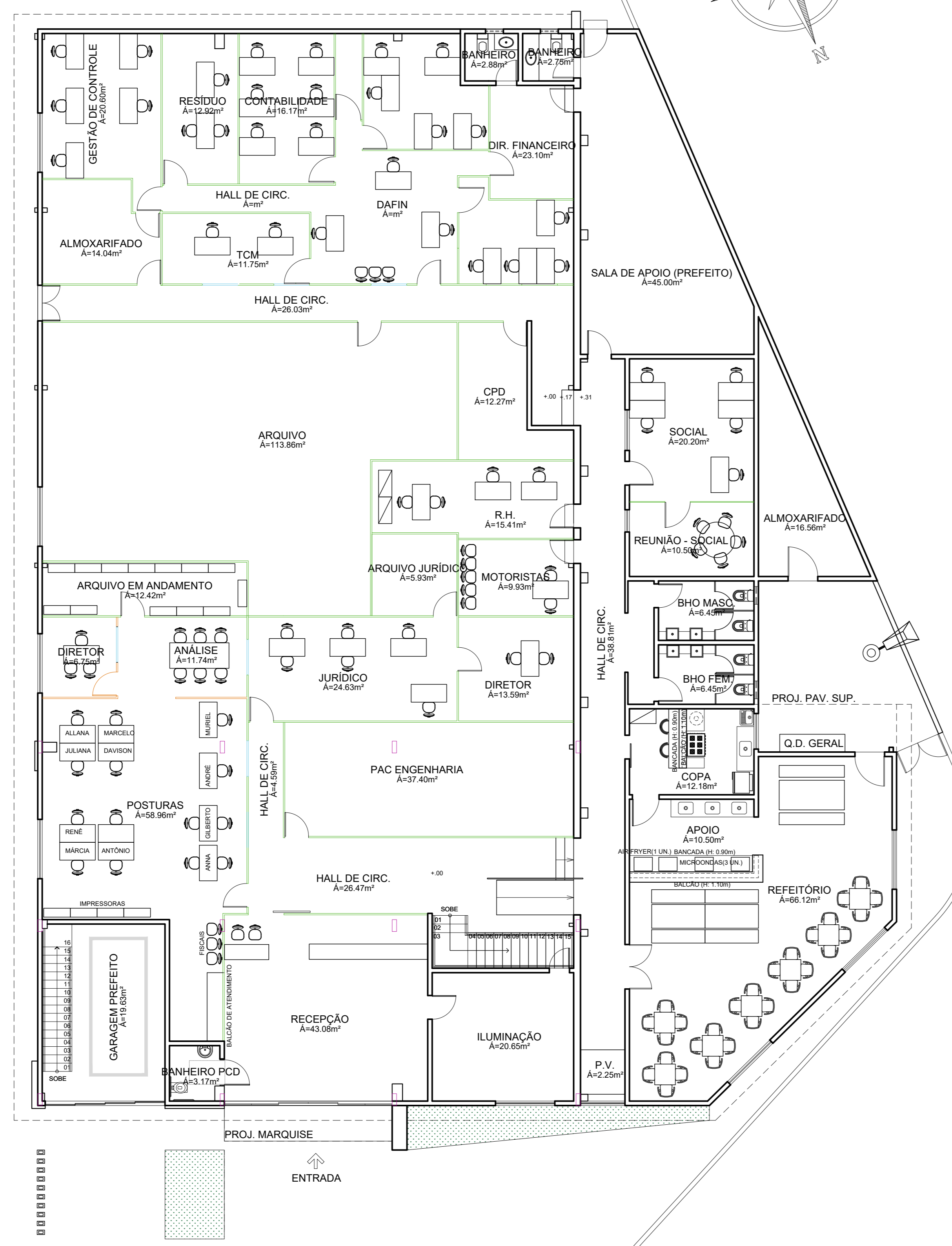
LAYOUT SESAN - PAV. TÉRREO ESC.: 1/100
