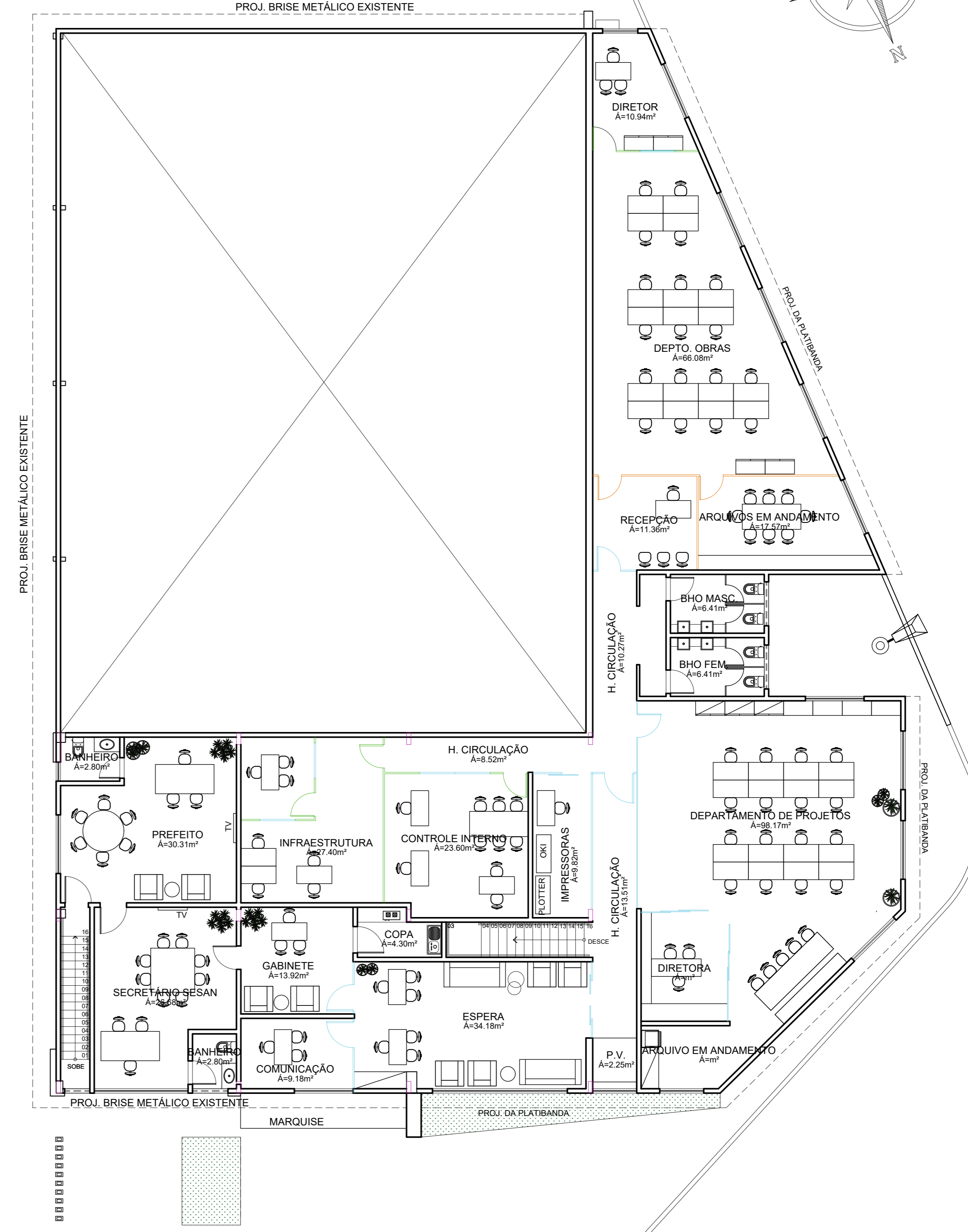
LAYOUT SESAN - PAV. SUPERIOR ESC.: 1/100
