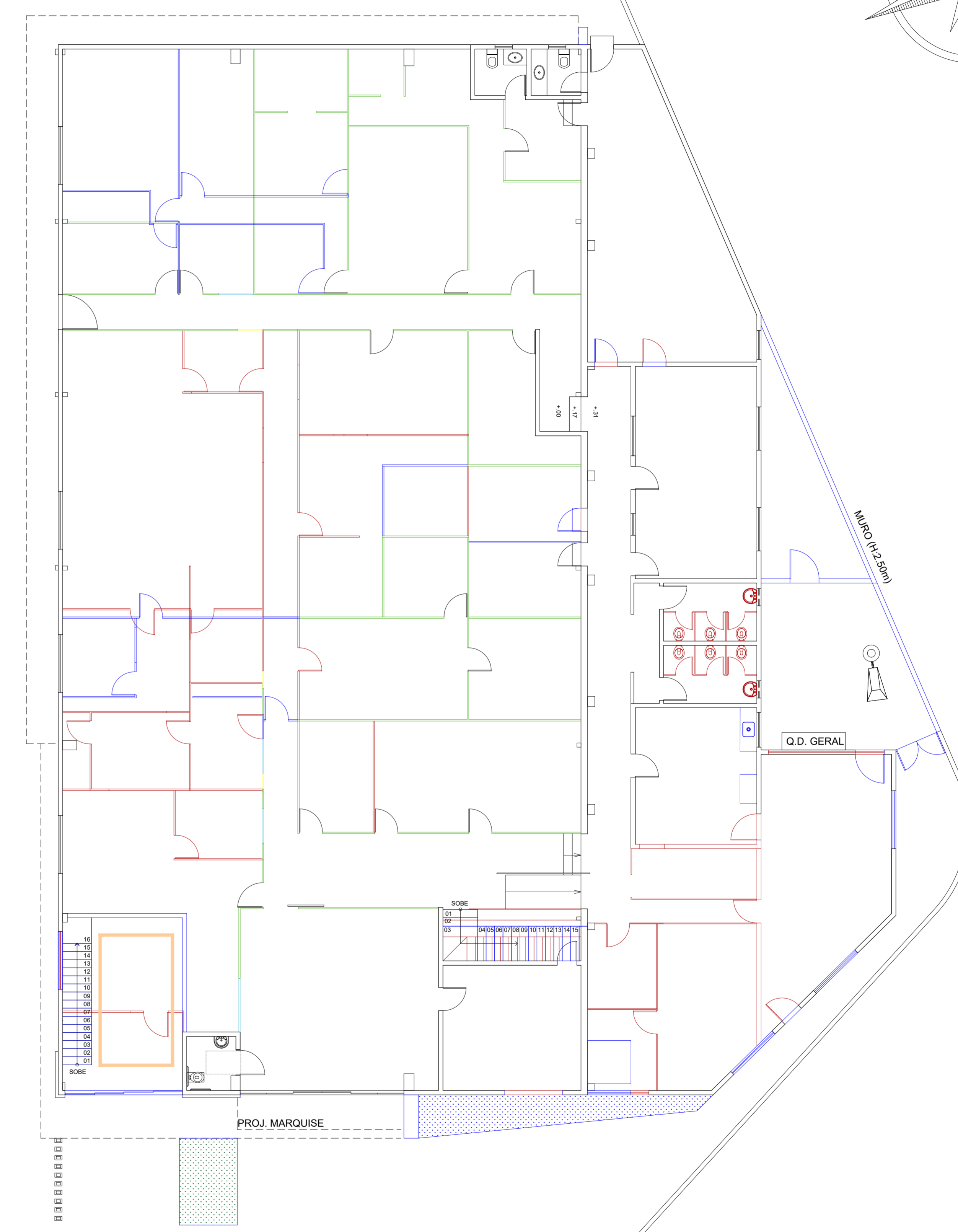
PLANTA DE REFORMA ESC.: 1/100
