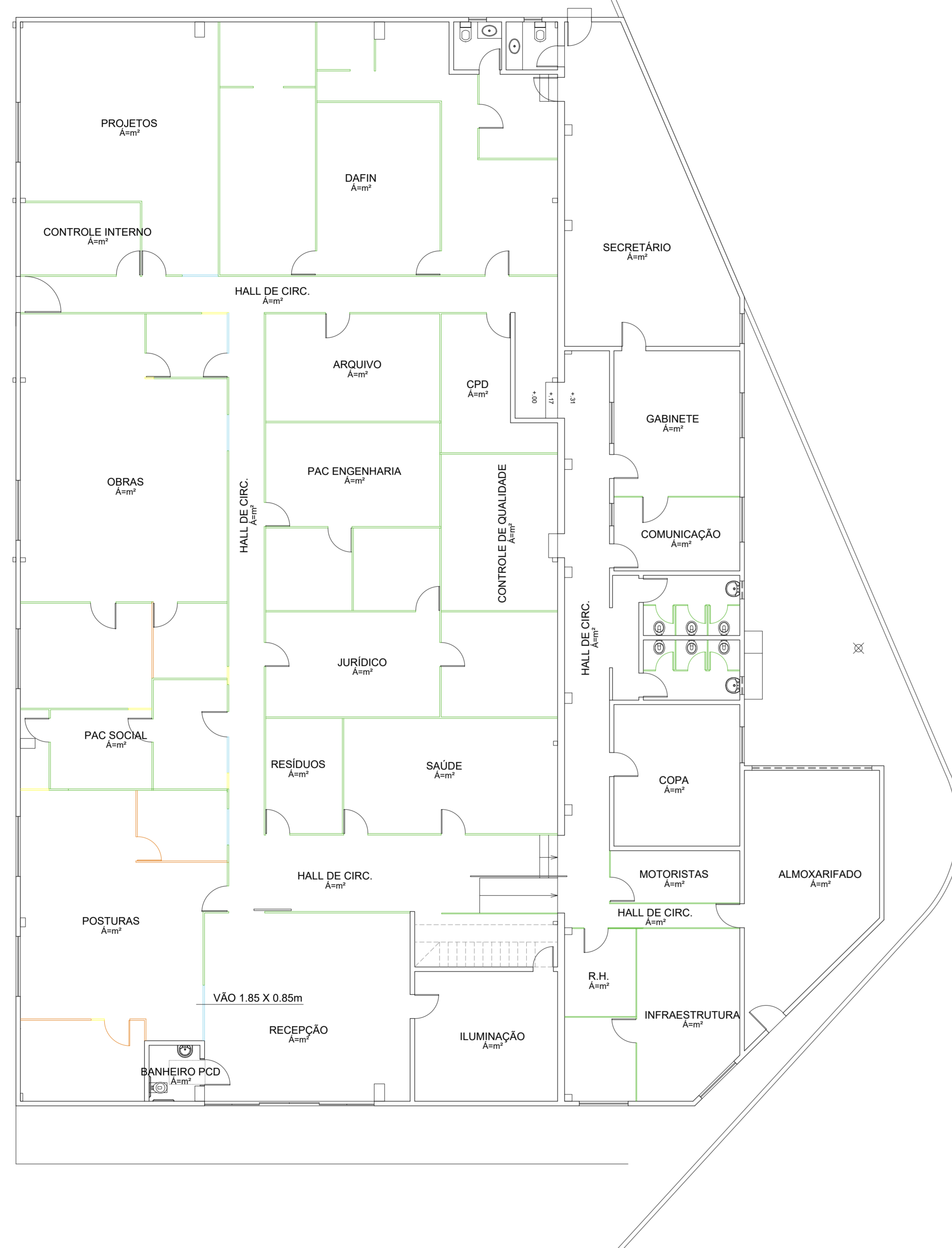
PLANTA BAIXA - SESAN ATUAL ESC.: 1/100
