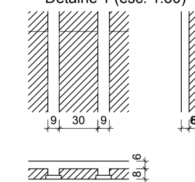
Detalhe 1 (esc. 1:30)
