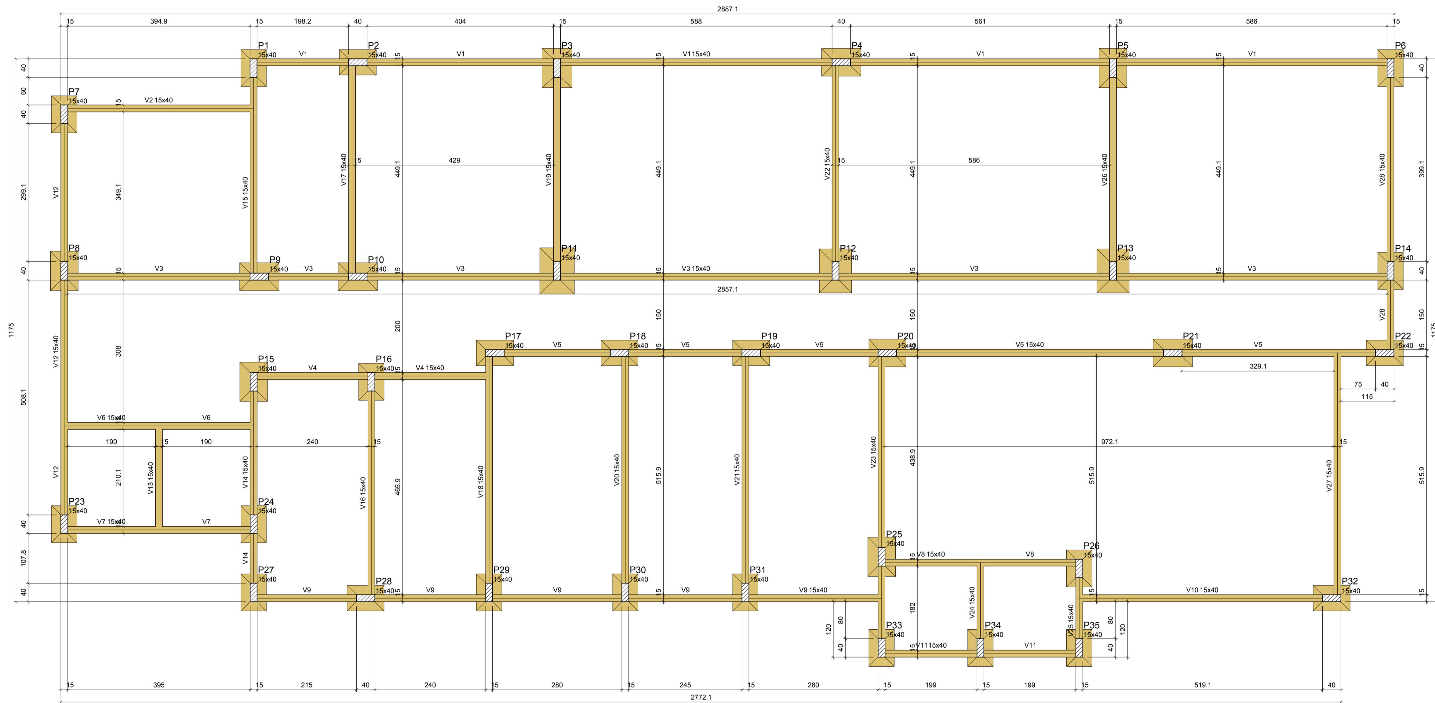
Forma do pavimento FUNDAC (Nível 0) escala 1:50
