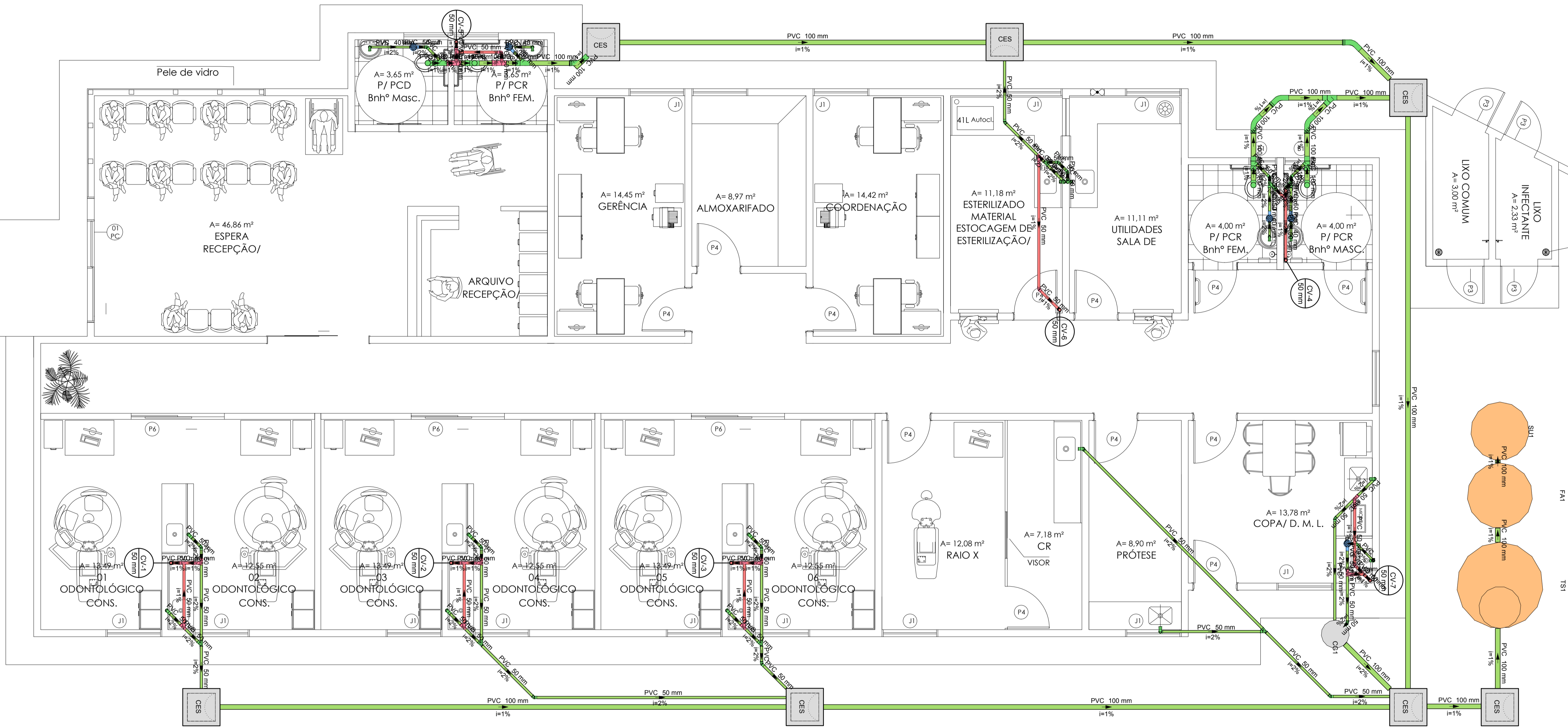
PLANTA BAIXA - TÉRREO ESCALA: 1:50
