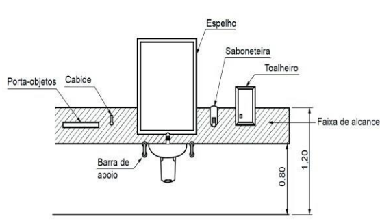
Figura 121 – Faixa de alcance de acessórios junto ao lavatório – Vista frontal
