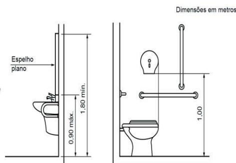
Figura 124 – Localização da papelreira de sobrepor (rolo) – Vista lateral
