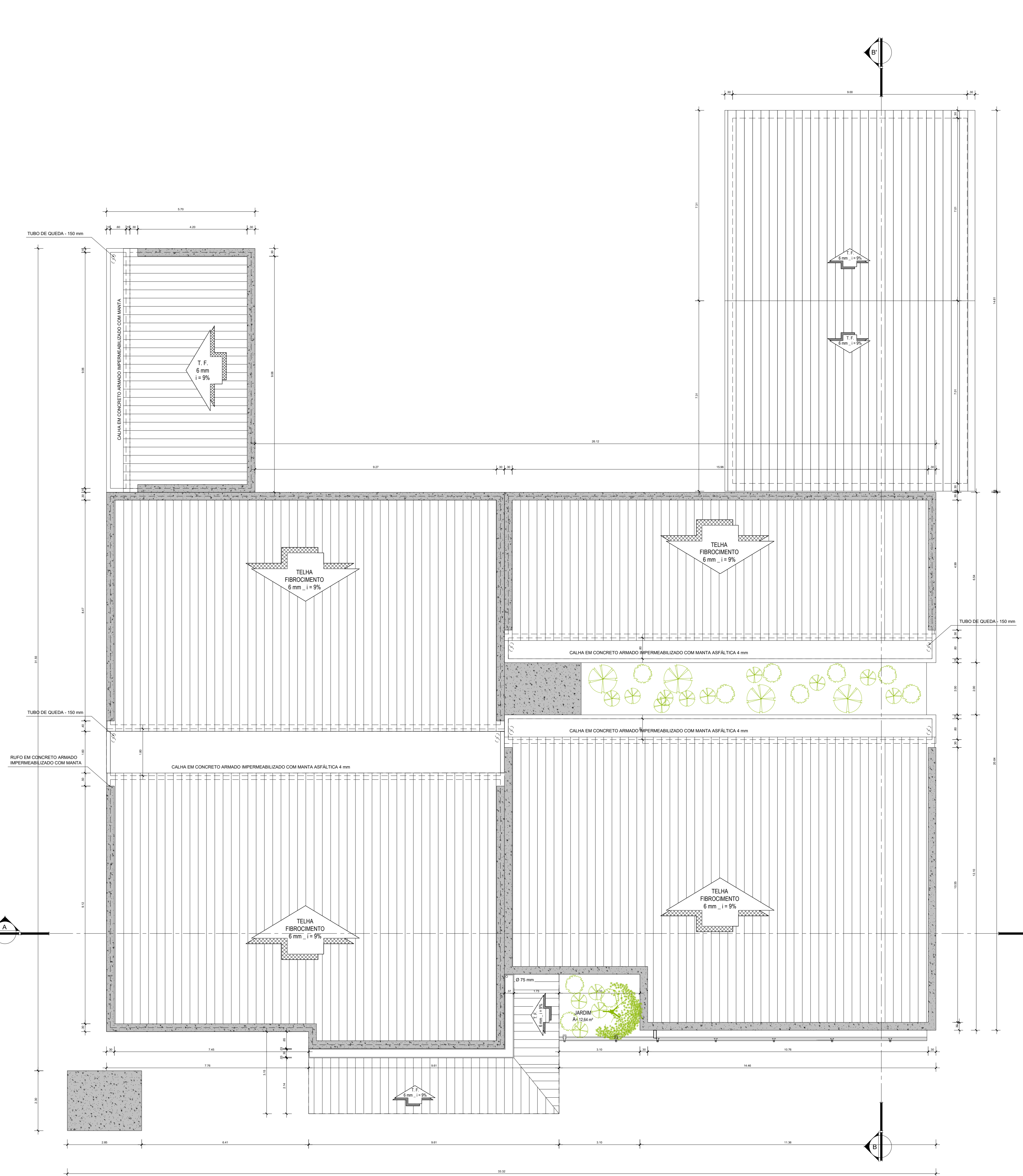
PLANTA DE COBERTURA ESC. 1:75
